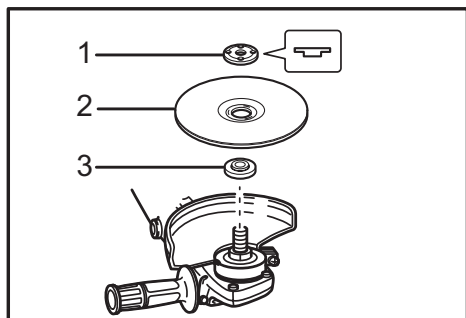
► 1. Contratuercas 2. Disco para esmerilar de centro hundido / multidisco 3. Brida interior
