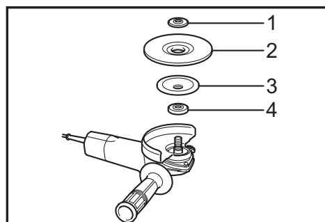
► 1. Contre-écrou 2. Meule flexible 3. Tampon d'appui 4. Bague interne
